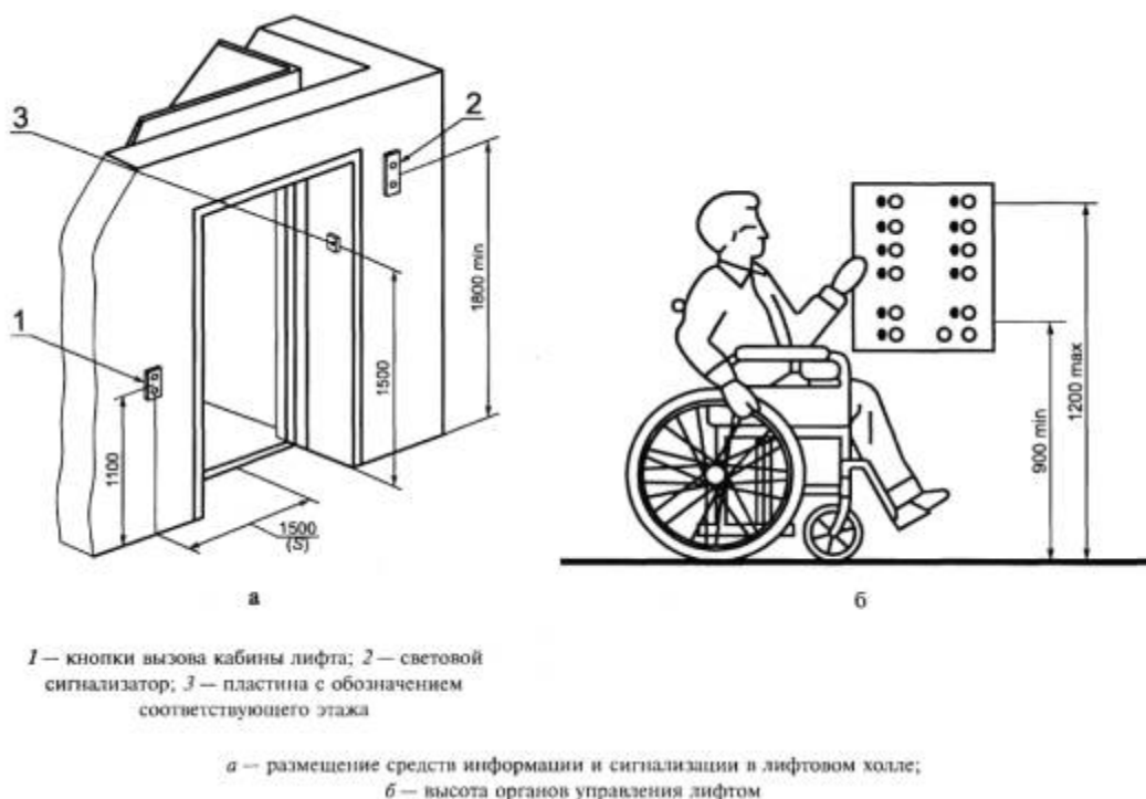
Рисунок 1-Средства информации и сигнализации в лифтах
